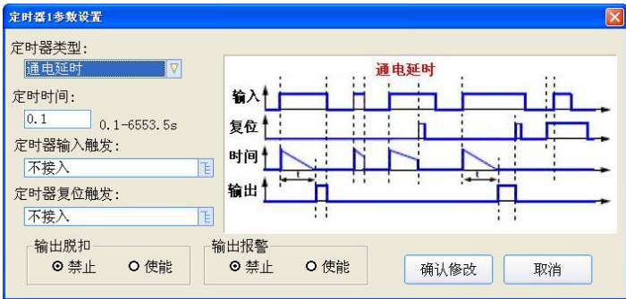
图 28 定时器
