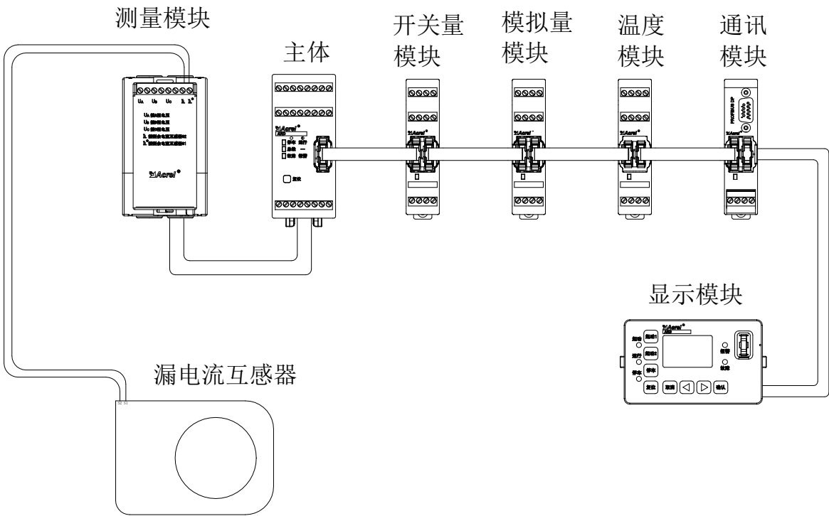
图 1 100A 及以下 ARD3SWT 产品组成（测量模块中带有电流互感器）
