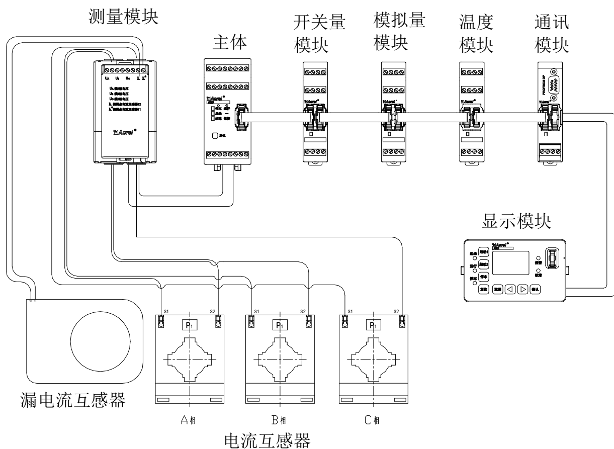
图 2 250A、800A ARD3SWT 产品组成
