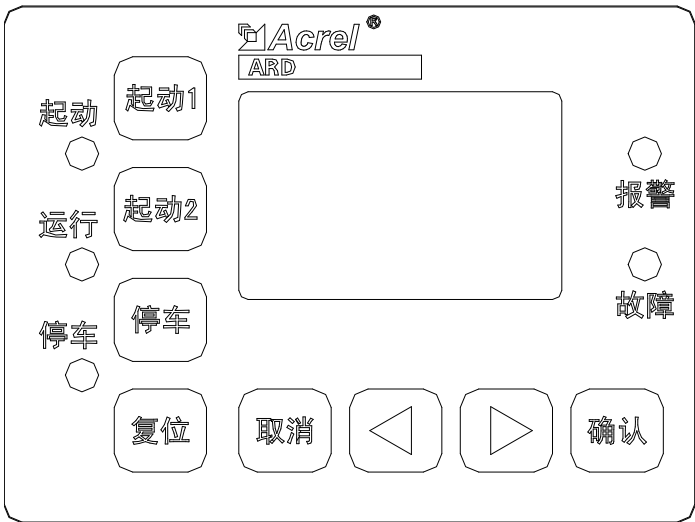
图 20 X60L 显示面板
