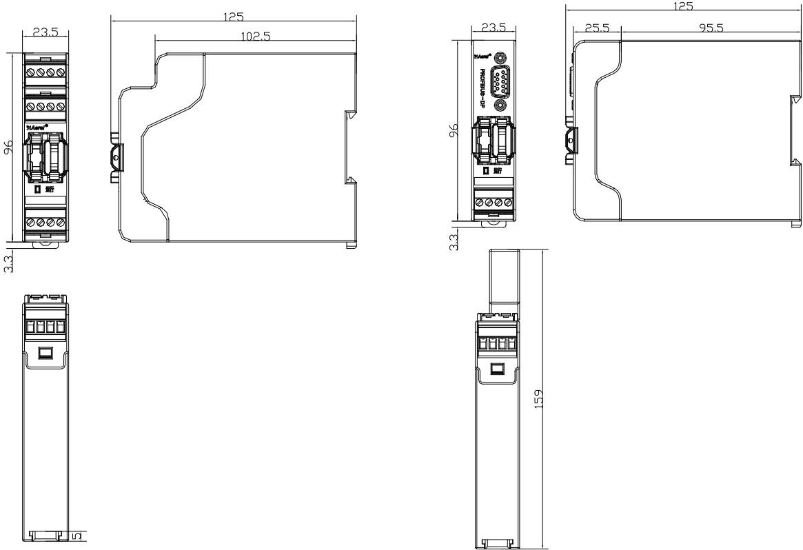
图 9 温度、模拟量、开关量外形尺寸
