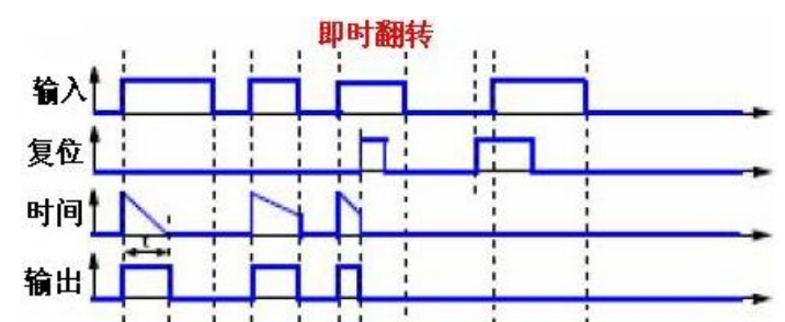
图 27 即时翻转定时器动作图
